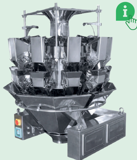
Dosificador por peso radial Diez cabezales - 10g a 3000g PARALLAX-1013
