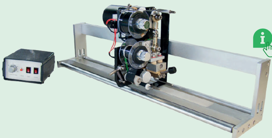
Codificador Hot Stamping Automático DAX-COD-HP450QT
