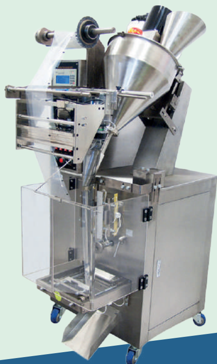
Máquinas Automáticas Verticales para Polvo (Envasado - Llenado - Sellado)
