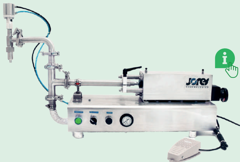
Dosificador de mesa con pistón para líquidos 100 ml - Baja viscosidad FP-100
