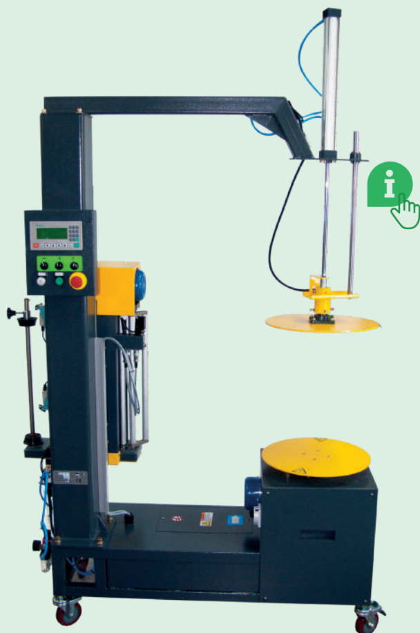
Máquina de envoltura elástica para cajas Con plato giratorio STR-6000
